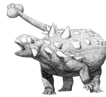
Euoplocephalus
