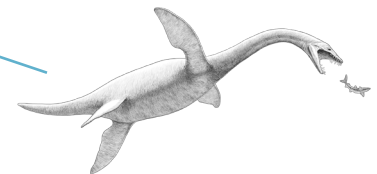
Plesiosaur
